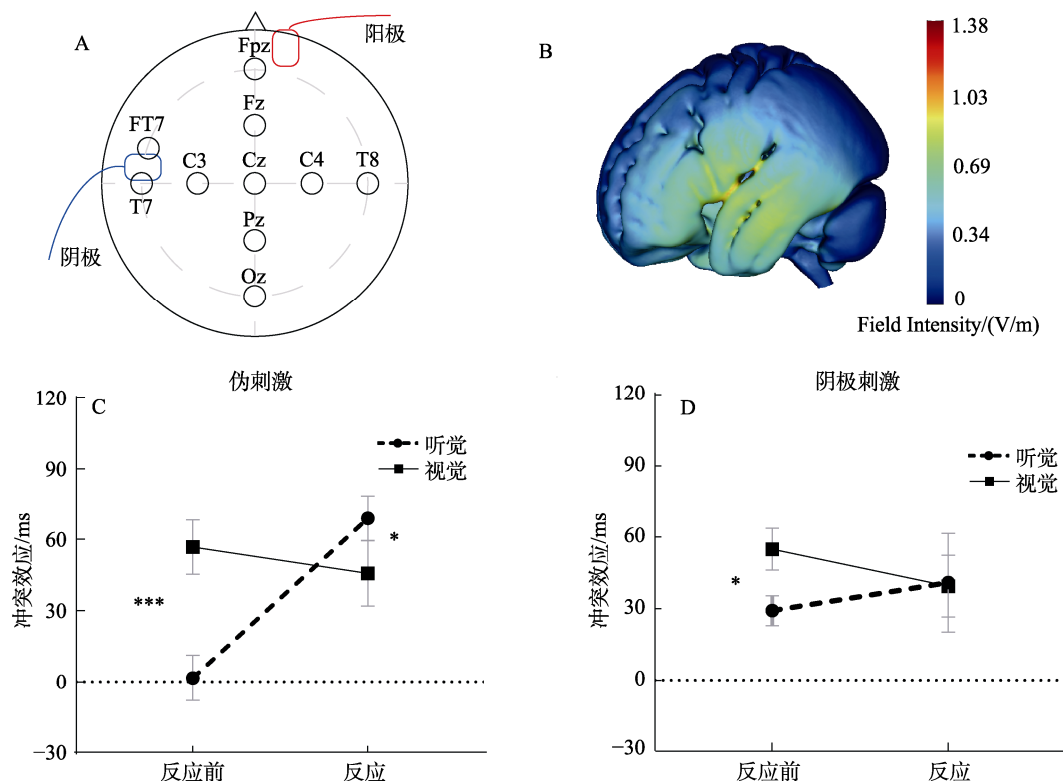
图3 A为左侧颞前叶皮层在国际 EEG 10-20 系统标准的定位示意图, 位于 T7 和 FT7 之间; B为 HD-explore 软件模拟左侧颞前叶皮层在标准脑模型中的电场模型; C为伪刺激条件下的实验结果; D为阴极刺激条件下的实验结果。
