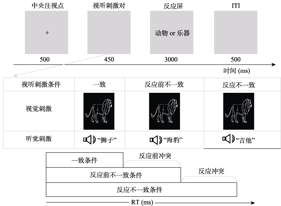
图 1 实验 1c 的刺激实例及实验流程图。视听刺激构成三种条件，一致条件：视听刺激完全一致；反应前不一致条件：视听刺激不一致但对应按键一致；反应不一致条件：视听刺激对应按键不一致。反应前冲突 = 反应前不一致条件的反应时 - 一致条件的反应时；反应冲突 = 反应不一致条件的反应时 - 反应前不一致条件的反应时。
