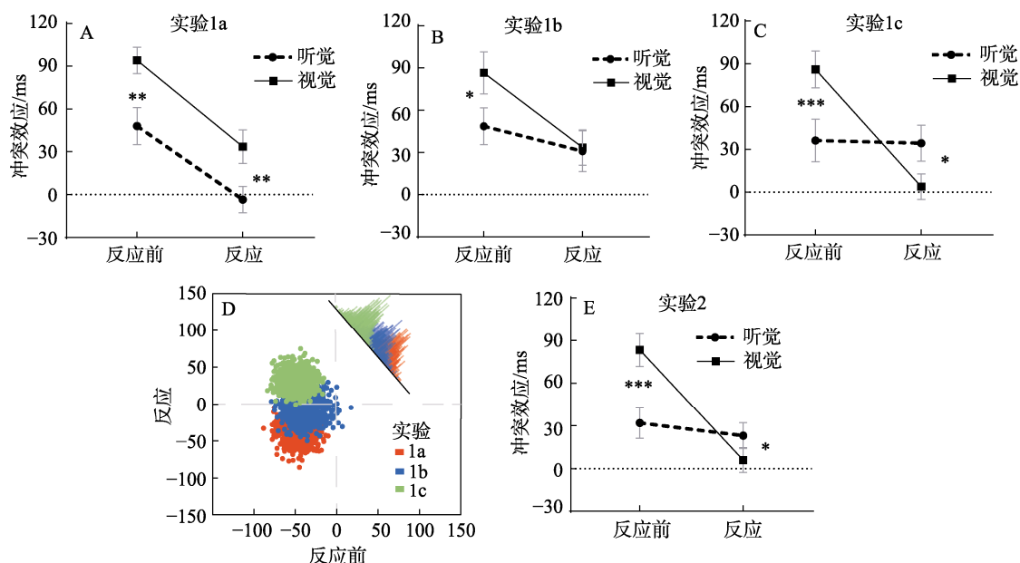
图2 实验1和2的结果图。A~C分别为实验1a~c的结果图; D为实验1每个实验的感觉主导指数(听觉冲突与视觉冲突之差)再抽样得到的样本均值分布图; E为实验2的结果图。
